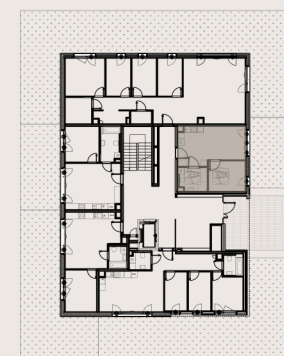
RZUT PARTERU BUDYNEK 1B
