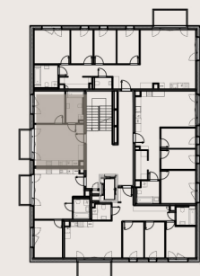
RZUT PIĘTRA 1 BUDYNEK 1B
