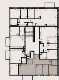
RZUT PIĘTRA 2 BUDYNEK 1B
