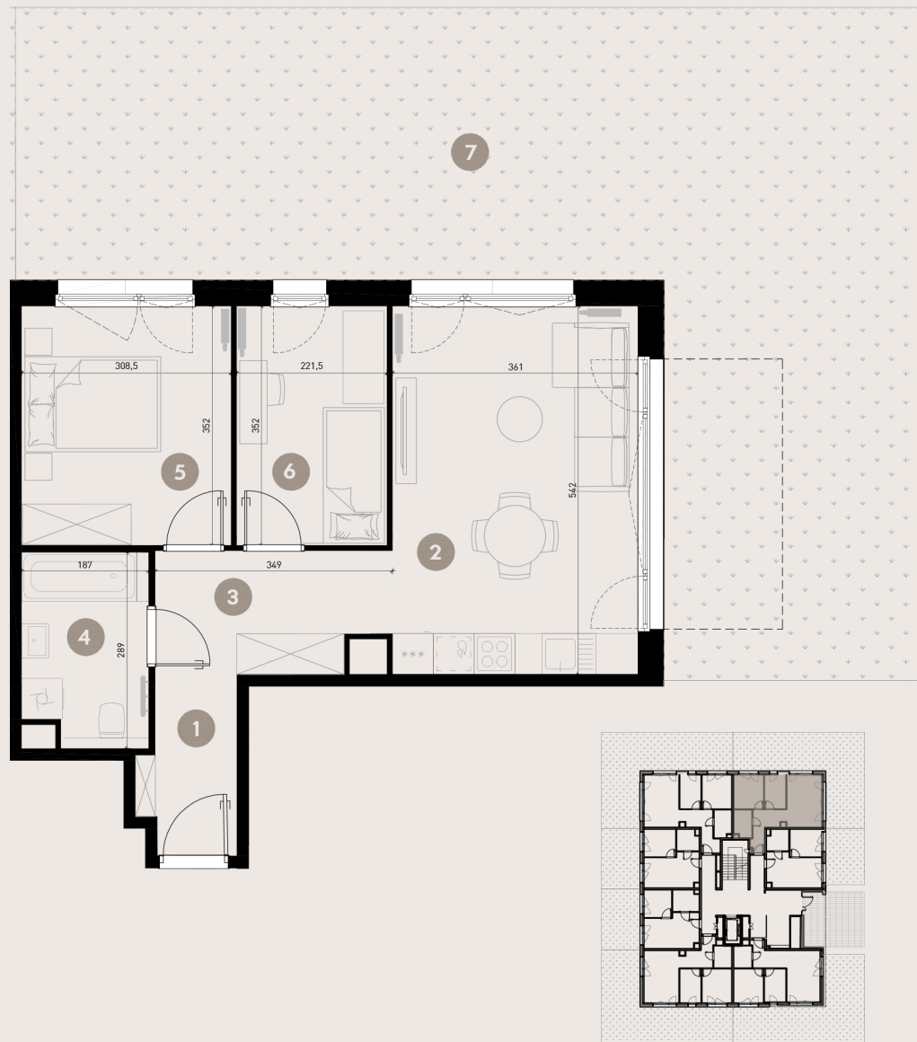
RZUT PARTERU BUDYNEK 1C
