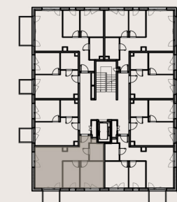
RZUT PIĘTRA 1 BUDYNEK 1C
