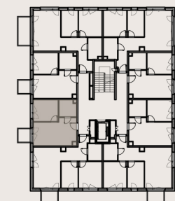
RZUT PIĘTRA 2 BUDYNEK 1C
