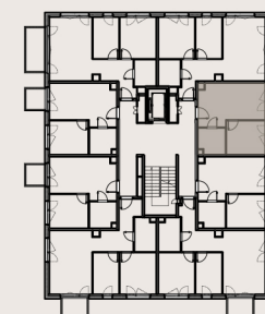
RZUT PIĘTRA 2 BUDYNEK 1D
